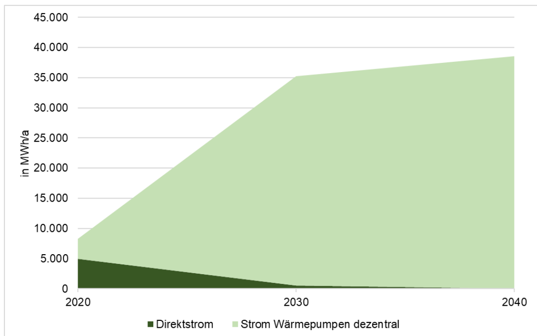
Abbildung 41: Zunahme des Strombedarfs durch Wärmerzeuger im Zielszenario
