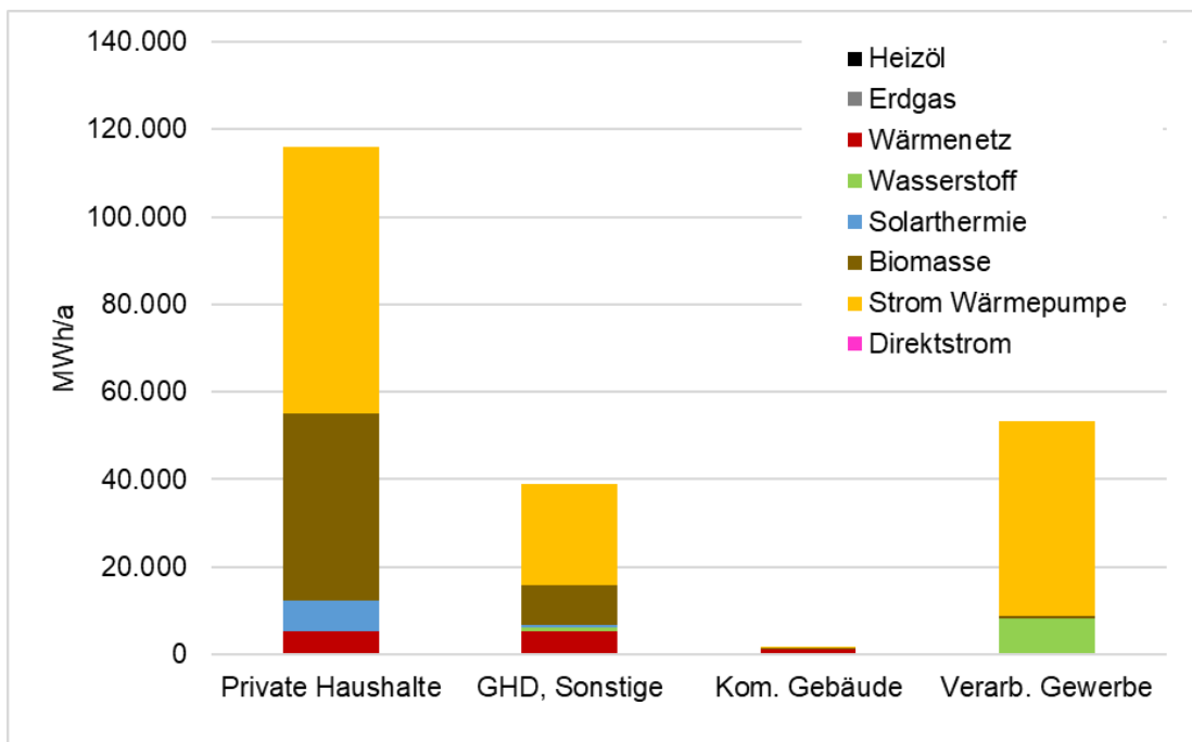
Abbildung 39: Wärmebedarf im Jahr 2040 nach Sektoren und Energieträgern
