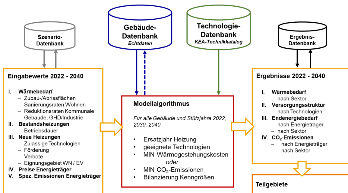
Abbildung 32: Modellstruktur
